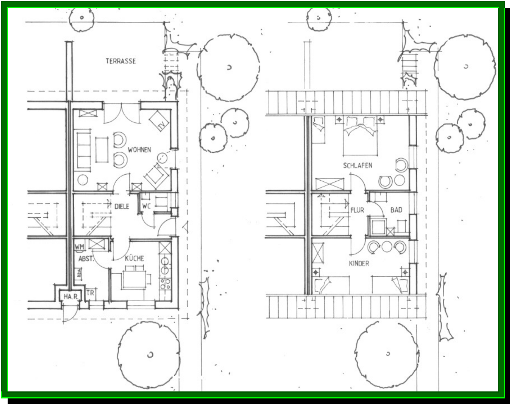
GRUNDRISS ERDGESCHOSS
